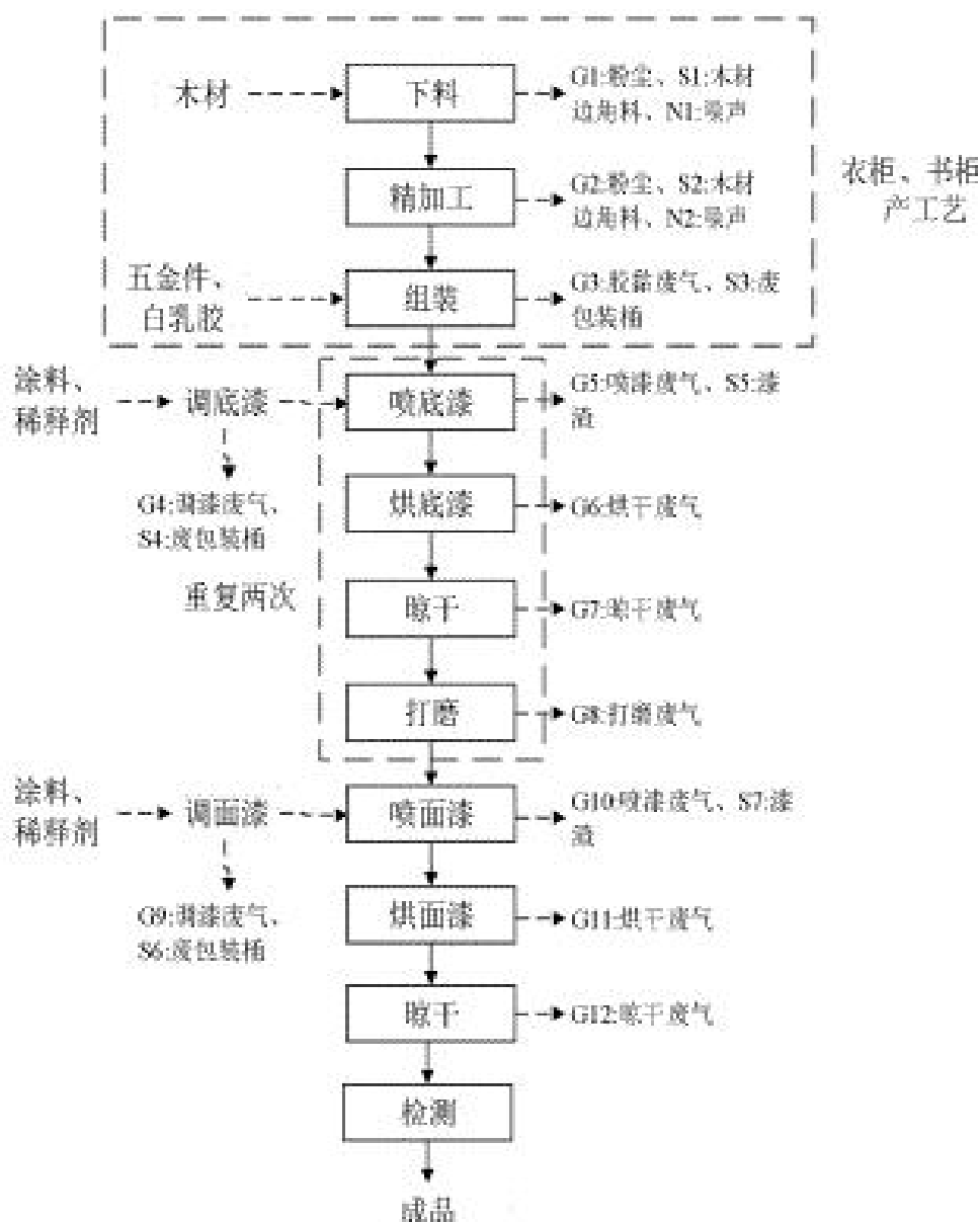
图1-3 生产工艺流程图
