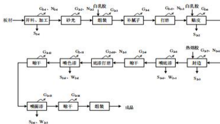
图 3-4 实木家具生产工艺流程图
