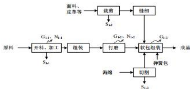
图 3-3 板式家具生产工艺流程图
