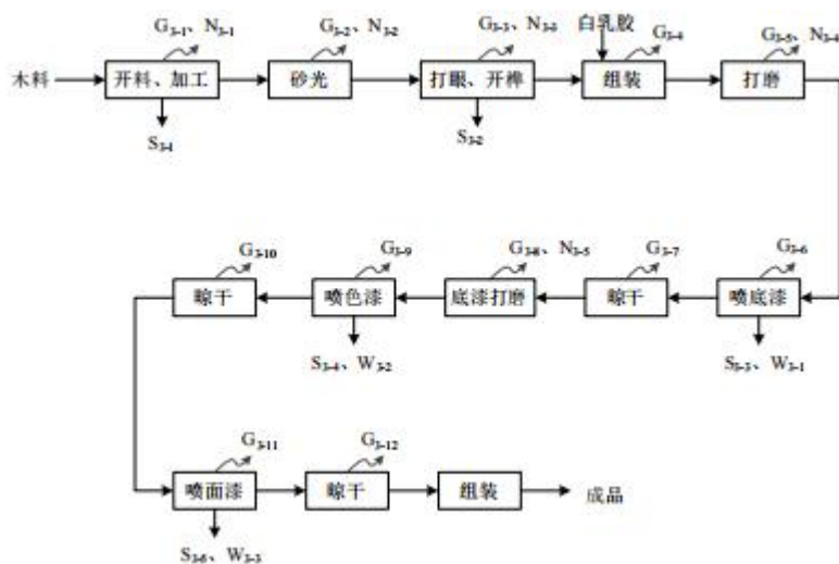
图 3-2 软包生产工艺流程图
